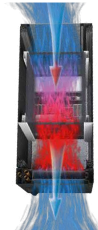
Luftstrom Serverrack m. Vertiv Knürr DCL (Schnittdarstellung)
