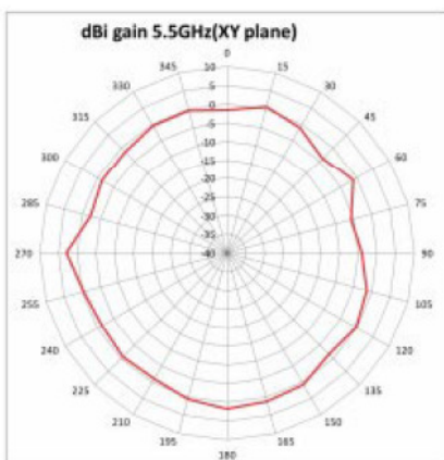
5-GHz-Antenne
